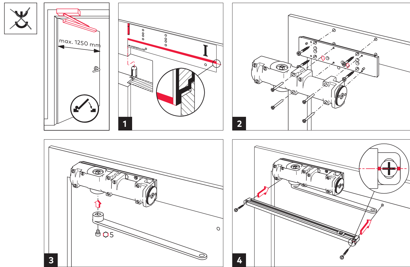
TS 93 B EN 1-5 WN 057113 45532 2020-04 5
