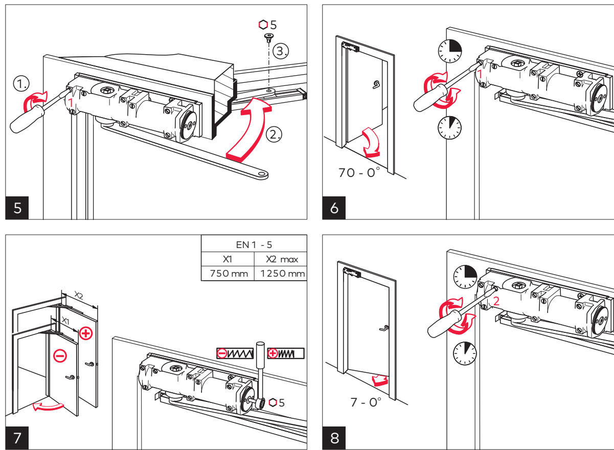
TS 93 B EN 1-5 WN 057113 45532 2020-04 6
